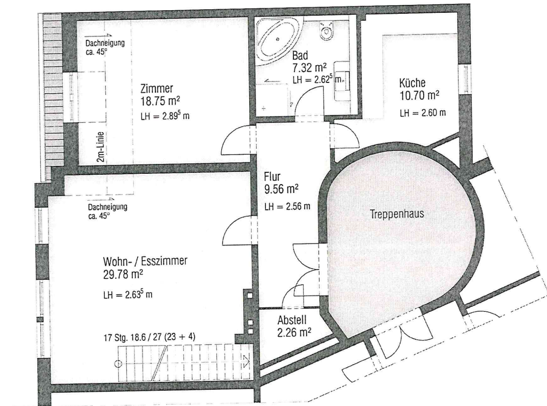
Grundriss 4. Obergeschoss M 1:100
