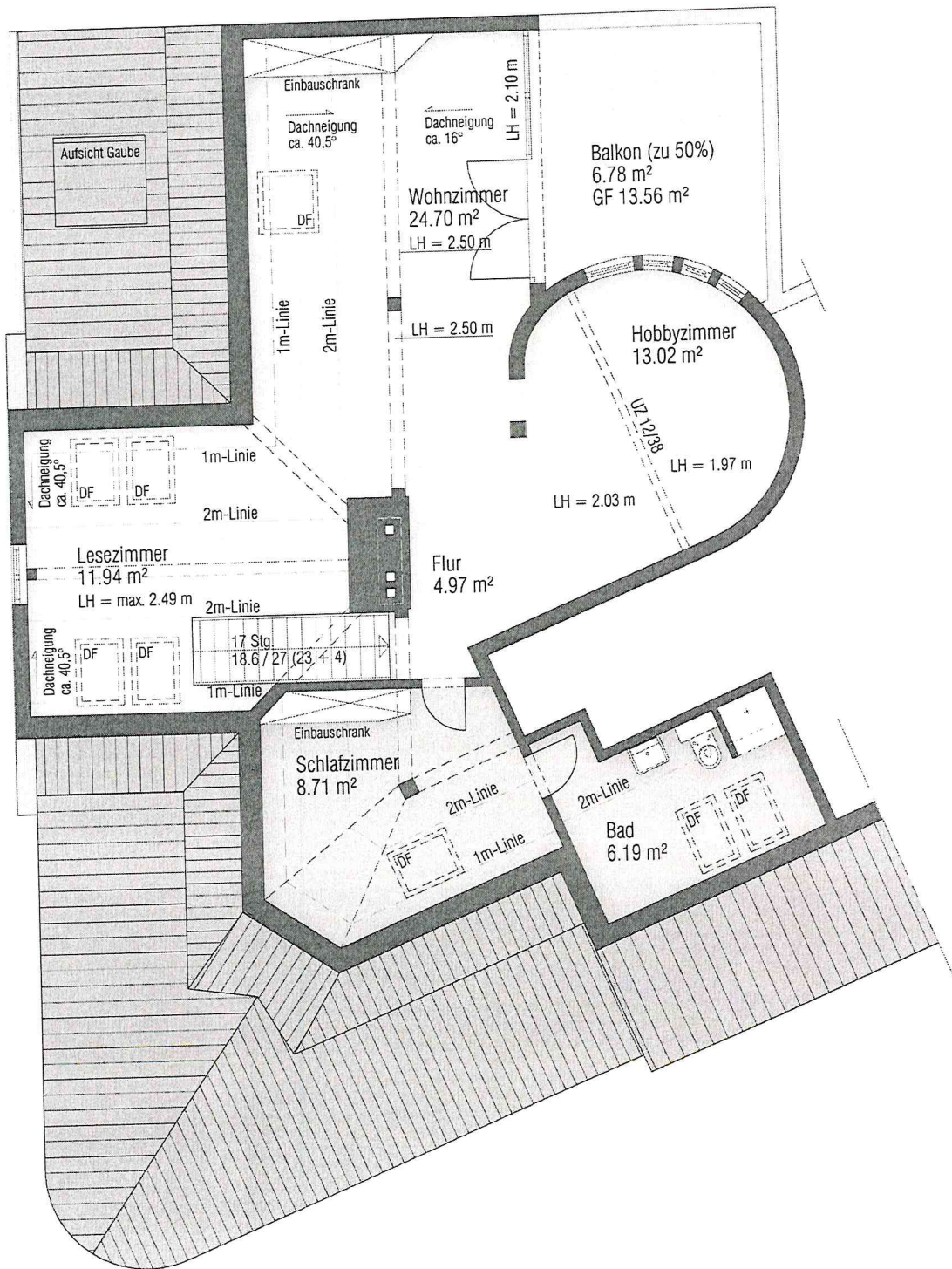
Grundriss Maisonettegeschoss M 1:100
